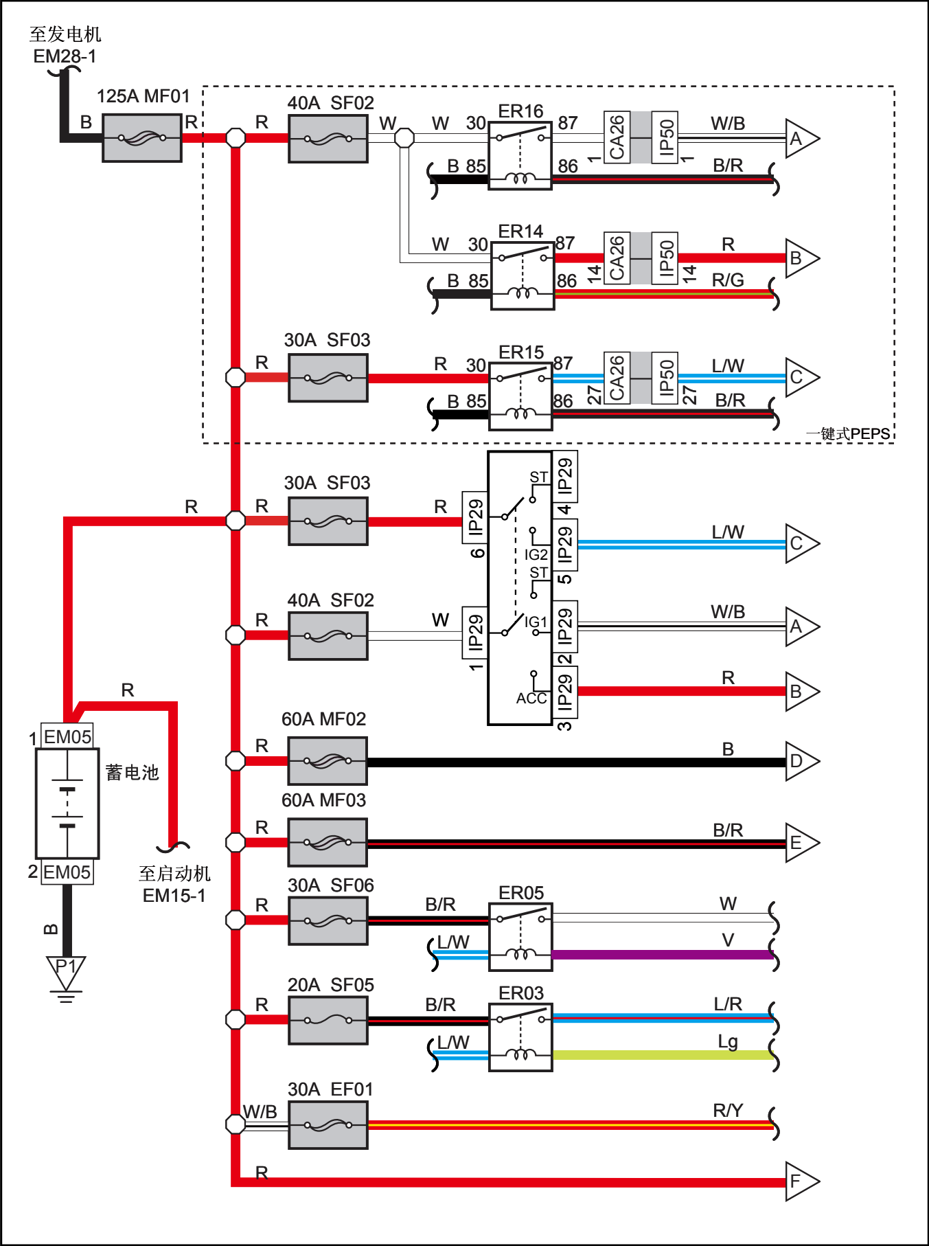
电源配电图1
